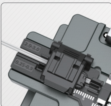
皮线
